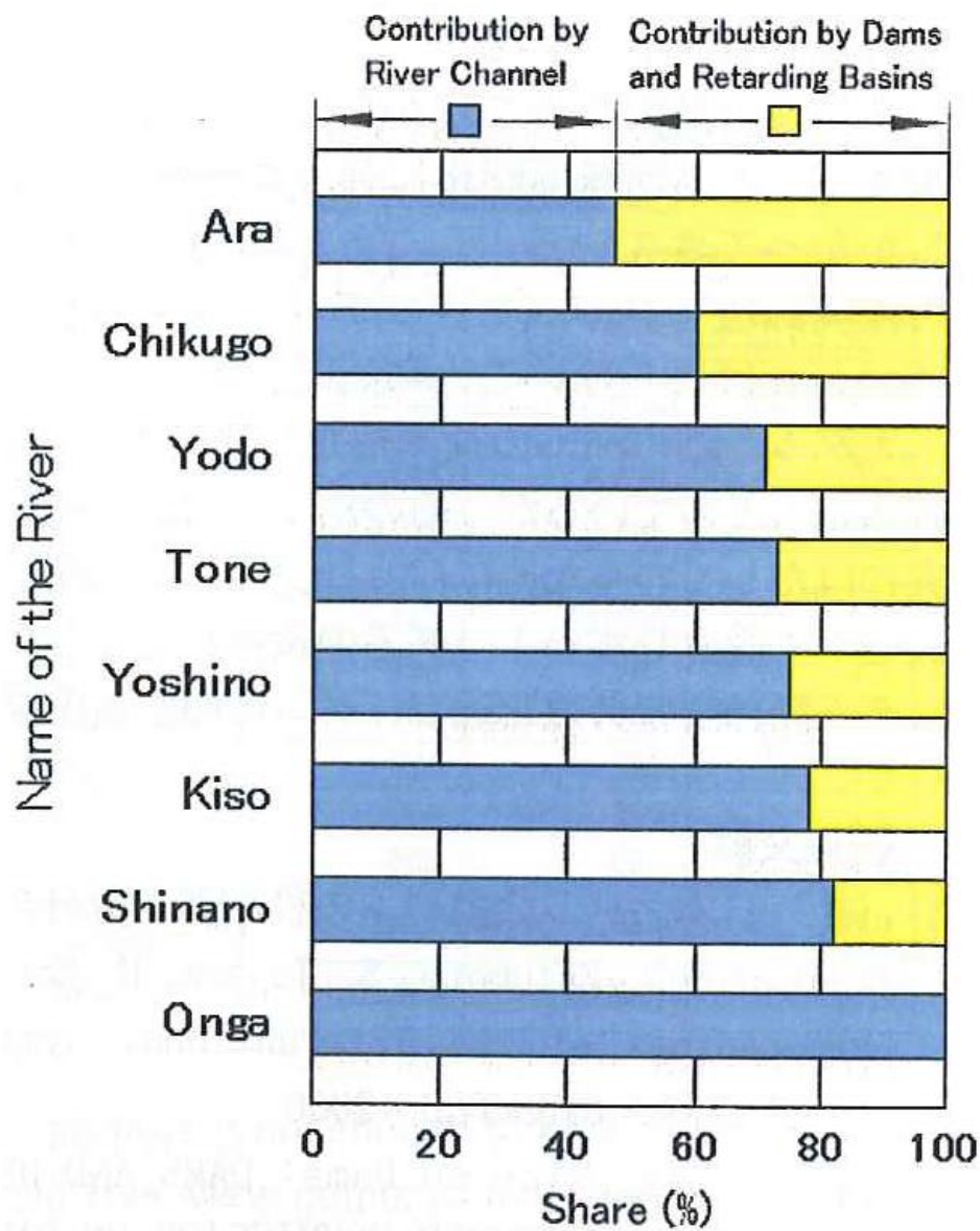
図-6 主要河川における河道・ダム等の洪水流量の分担率
