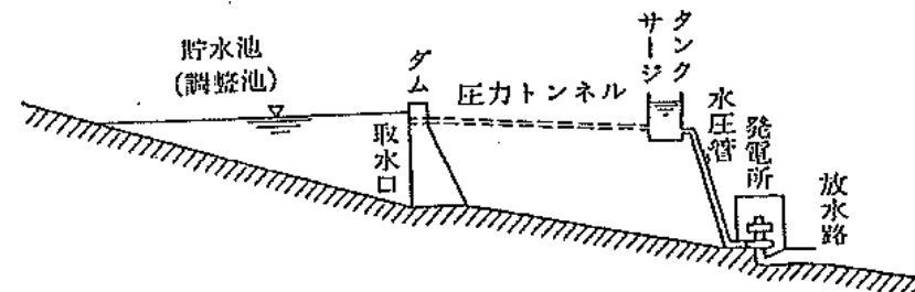
② ダム水路式
